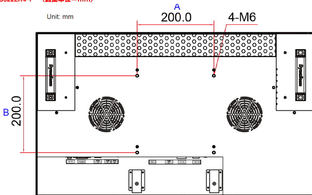
DS322LR4-1 (図面単位=mm)
